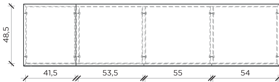
PIANTA | PLAN
